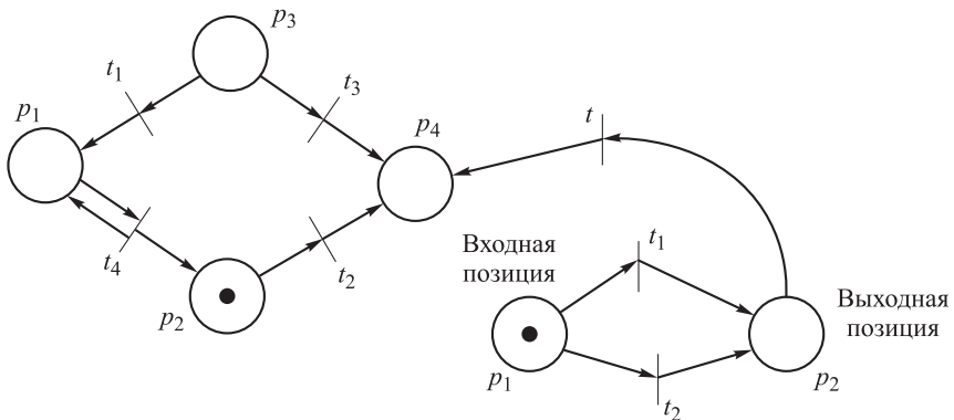
Рис. 4. Структурированная сеть Петри
