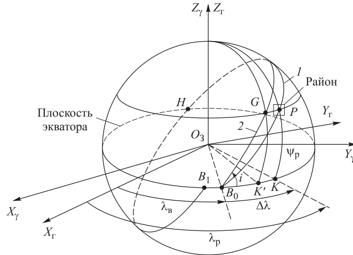
Рис. 1. Трассы полета КА в нормальном гравитационном поле Земли (1) и по оскулирующей орбите (2)
