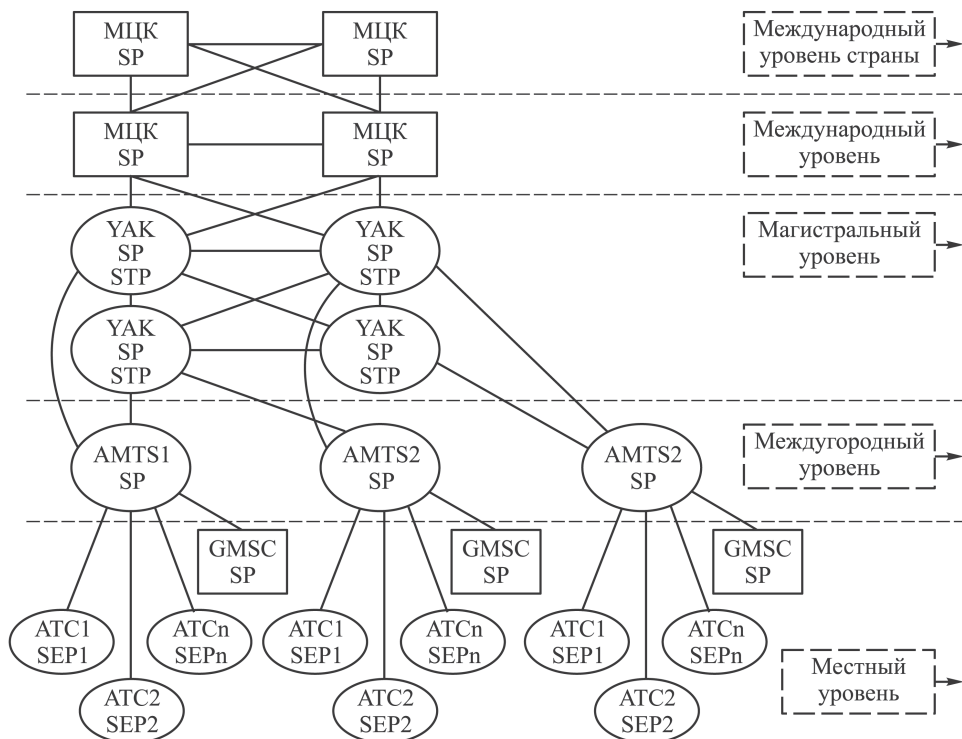
Рис. 2. Архитектура системы ОКС-7 сети ТфОП/ISDN, обеспечивающая сигнализацию в сети GSM
