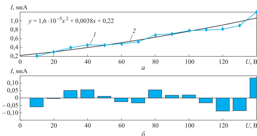
Рис. 2. Квадратичная математическая модель статической вольт-амперной характеристики ППКЧД (а) и погрешность этой модели (б)
